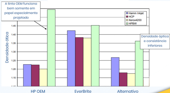
Densidade óptica da tinta preta nos papéis - HP56
